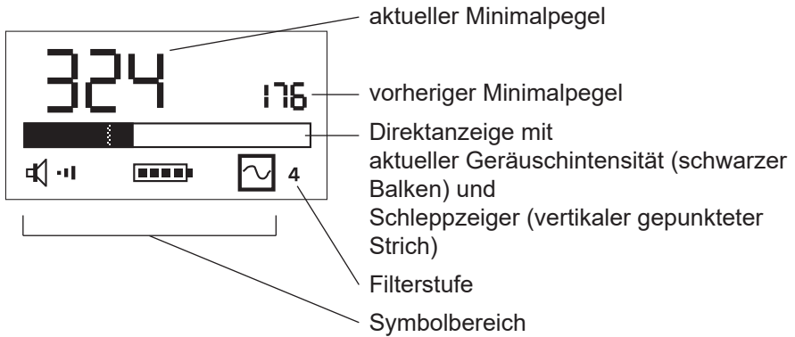
Abb. 2: AquaTest T10 – Display im Arbeitsbereich Betrieb
