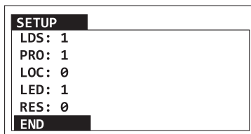
Fig. 8: Menu SETUP (domaine de travail Réglages de base )
