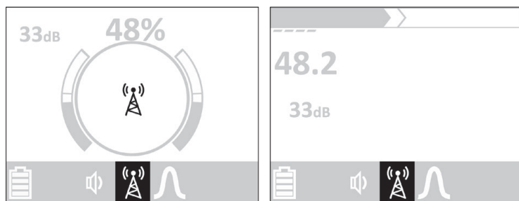
Fig. 27: Écran du récepteur – Localisation passive en mode Radio Image de gauche : Interface utilisateur UtiliGuard2 Image de droite : Interface utilisateur Classique
