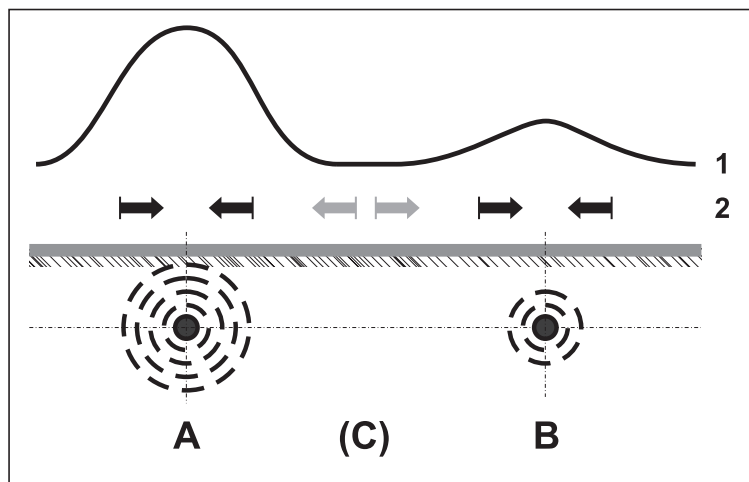
Fig. 28: Situation de localisation en cas de conduites rapprochées
