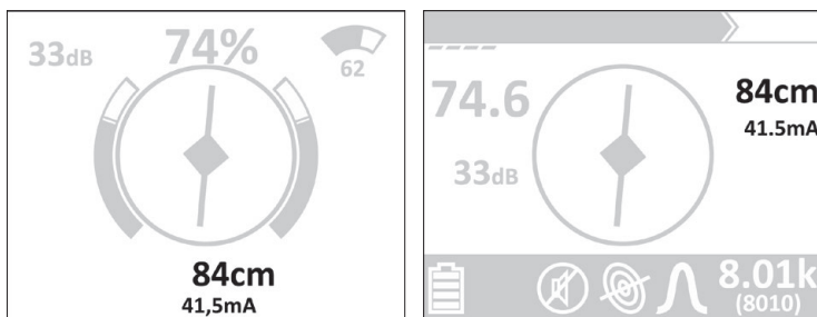
Fig. 9: Écran du récepteur - Affichage de la profondeur ( ici : profondeur 84 cm, intensité 41,5 mA) Image de gauche : Interface utilisateur UtiliGuard2 Image de droite : Interface utilisateur Classique
