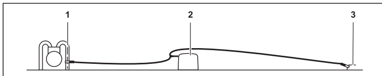
Fig. 22: Agencement des appareils pour l'injection directe
