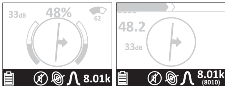
Fig. 10: Écran du récepteur – Barre d'outils Image de gauche : Interface utilisateur UtiliGuard2 Image de droite : Interface utilisateur Classique
