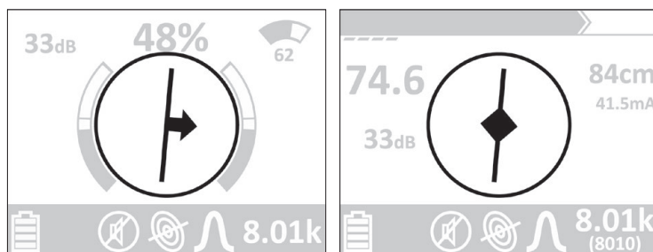
Fig. 6: Écran du récepteur - Boussole
