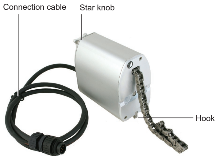
Fig. 15: Striker
