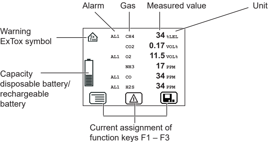
Fig. 2: Multitec 520 display
