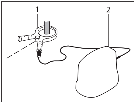
Abb. 26: Anordnung der Geräte beim Besenden mit Anlegezange 1 Anlegezange 2 Generator
