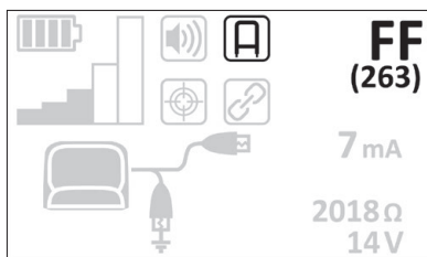
Abb. 33: Display des Generators – Schrittspannungssonde angeschlossen (hier: Symbol Schrittspannungssonde , FF (263))
