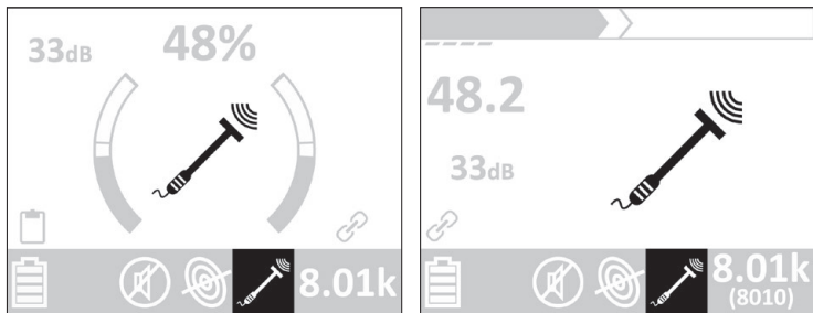
Abb. 40: Display des Empfängers – Empfangsantenne angeschlossen
