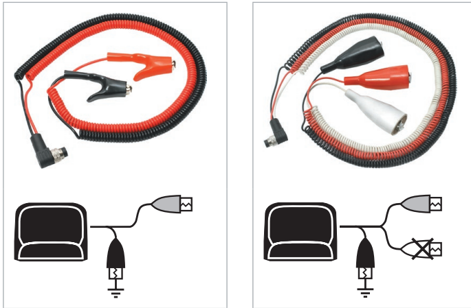
Abb. 23: Kabelsätze (oben) und zugehörige Symbole (unten)
