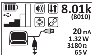
Abb. 15: Display des Generators – Sendebetrieb
