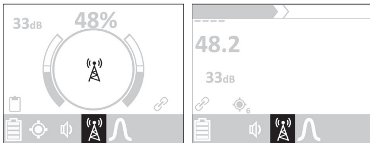
Abb. 30: Display des Empfängers – Passive Ortung im Ortungsmodus
