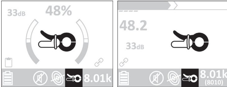
Abb. 39: Display des Empfängers – Empfangszange angeschlossen
