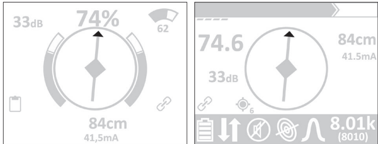
Abb. 27: Display des Empfängers – Richtungserkennung (Pfeil an Kompassnadel)
