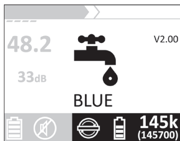
Abb. 36: Display des Empfängers – Markerball-Antenne angeschlossen ( hier : Frequenz 145 kHz / Symbol Wasser , Marker-Wahl Automatisch , Softwareversion V2.00) Die Ansicht ist für beide Nutzer-oberflächen identisch.
