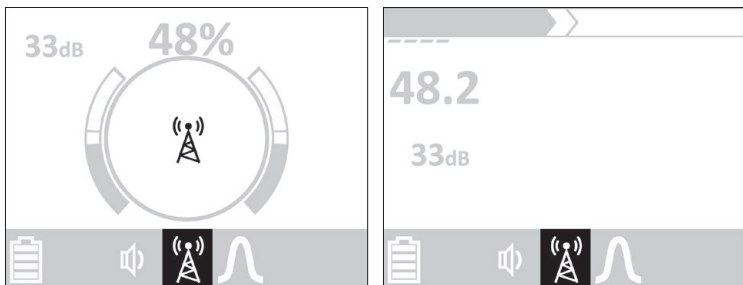
Abb. 27: Display des Empfängers – Passive Ortung im Ortungsmodus Radio Bild links: Nutzeroberfläche UtiliGuard2 Bild rechts: Nutzeroberfläche Klassisch
