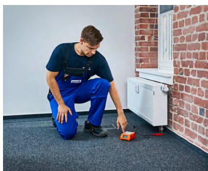
Escuta de uma tubagem com um recetor AF 50 e um gerador FG 50
