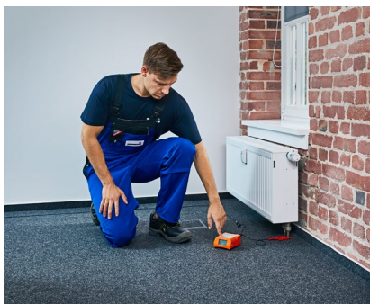
Besenden einer Leitung mit dem Empfänger AF 50 und dem Generator FG 50
