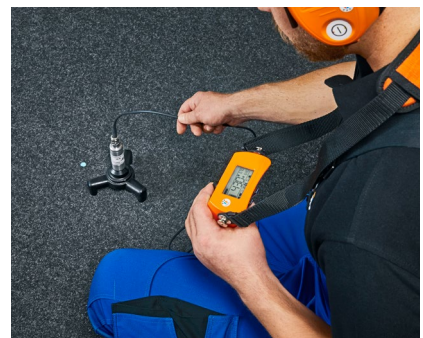
Leckageortung mit dem Empfänger AF 50 und dem Universalmikrofon UM 50
